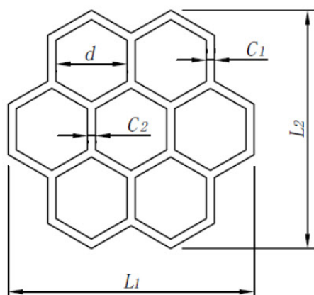
图 8 常用梅花管断面结构示意图
