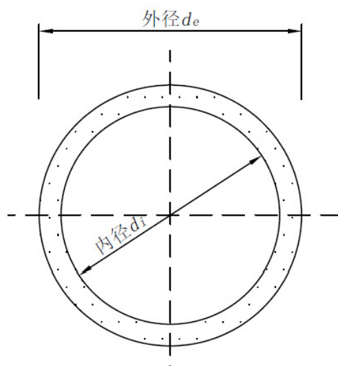
图 5 实壁管断面结构示意图
