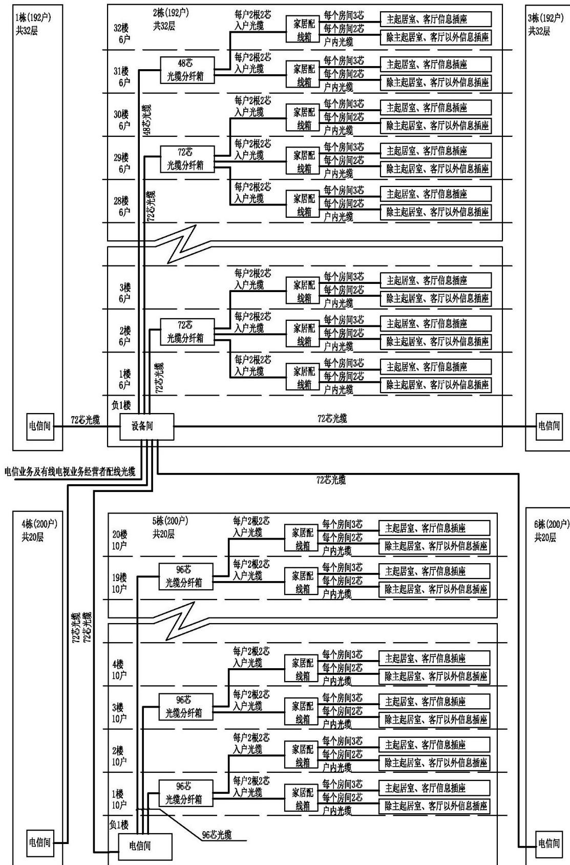
图 1 高层住宅纤芯方案示例图
