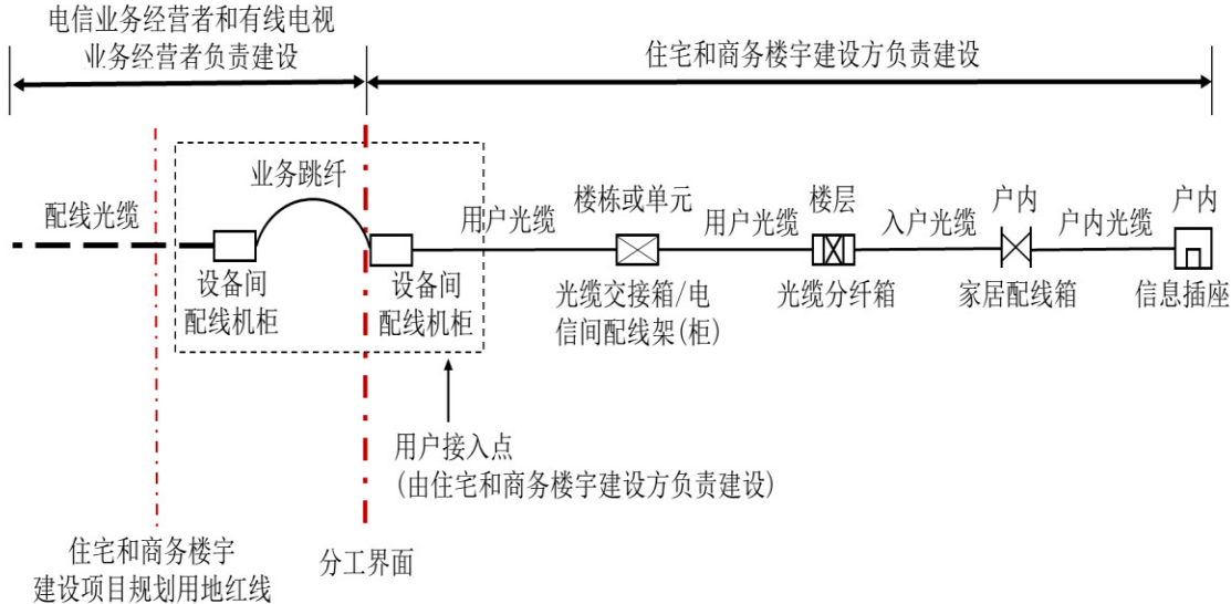
图 3.1.3 光纤到户工程网络建设分工界面图
